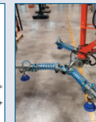
MANIPOLATORE AZZERATORE DI PESO
