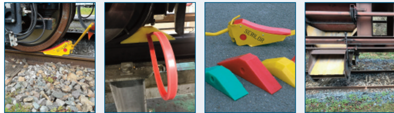
CUNEI FERROVIARI
